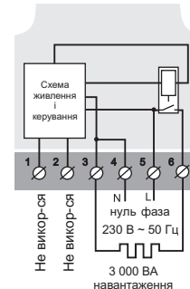
Схема 1. Спрощена внутрішня схема і схема підключення
