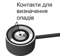
Рисунок 3. Розташування датчика опадів і нагрівального кабелю при підігріві ґрунту
